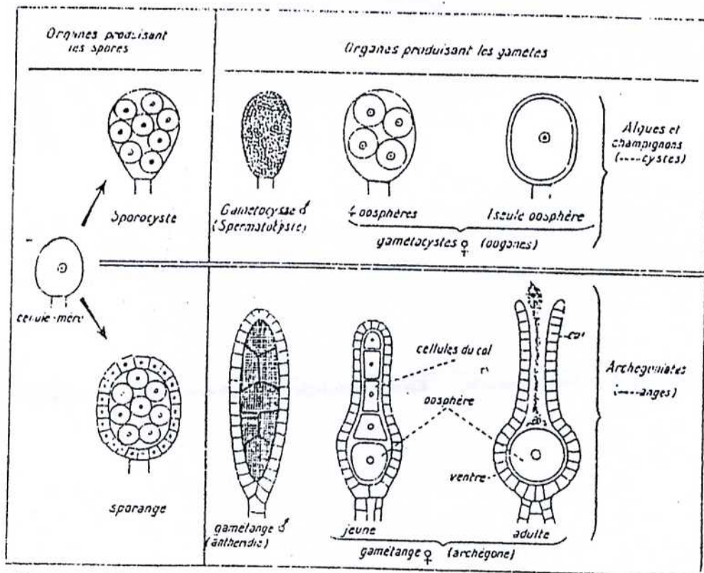
FIG. — Distinction entre les sporocystes et les gamétocystes des Algues et des Champignons et les sporanges et les gamétanges des Archégoniates.
